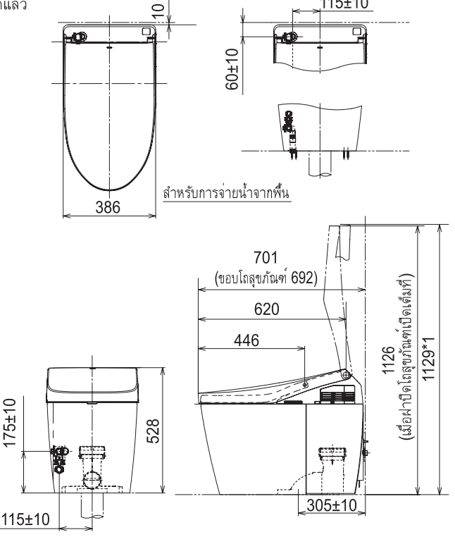
แผนภาพผลิตภัณฑ์ (ที่ติดตั้งเสร็จแล้ว)แบบ AH (หน่วย: มม.)
