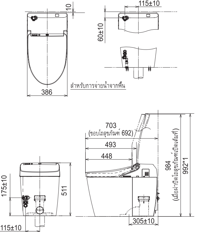
แผนภาพผลิตภัณฑ์ (ที่ติดตั้งเสร็จแล้ว)แบบ DH (หน่วย: มม.)
