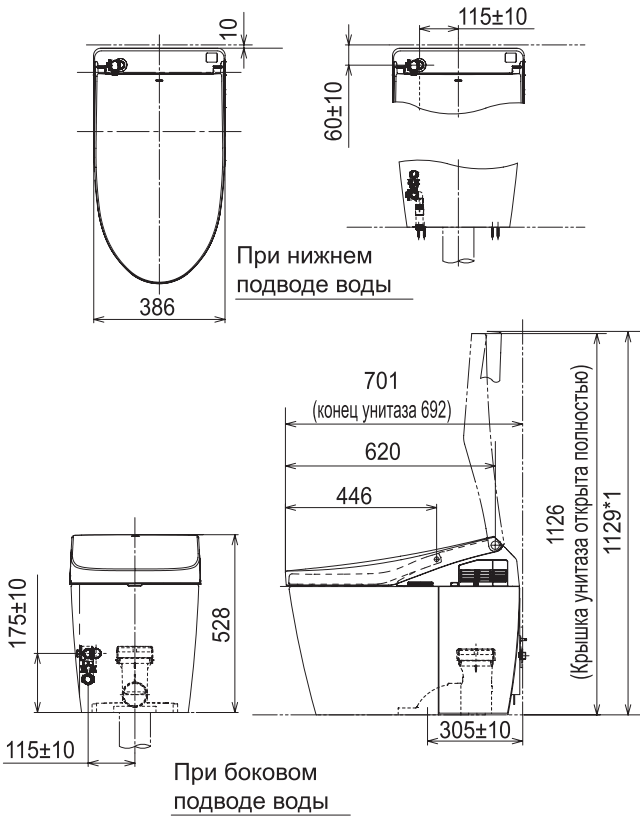
Чертеж изделия (по окончании монтажа) Модель АН (ед.: мм)
