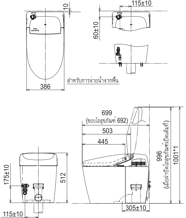
แผนภาพผลิตภัณฑ์ (ที่ติดตั้งเสร็จแล้ว)แบบ RH (หน่วย: มม.)
